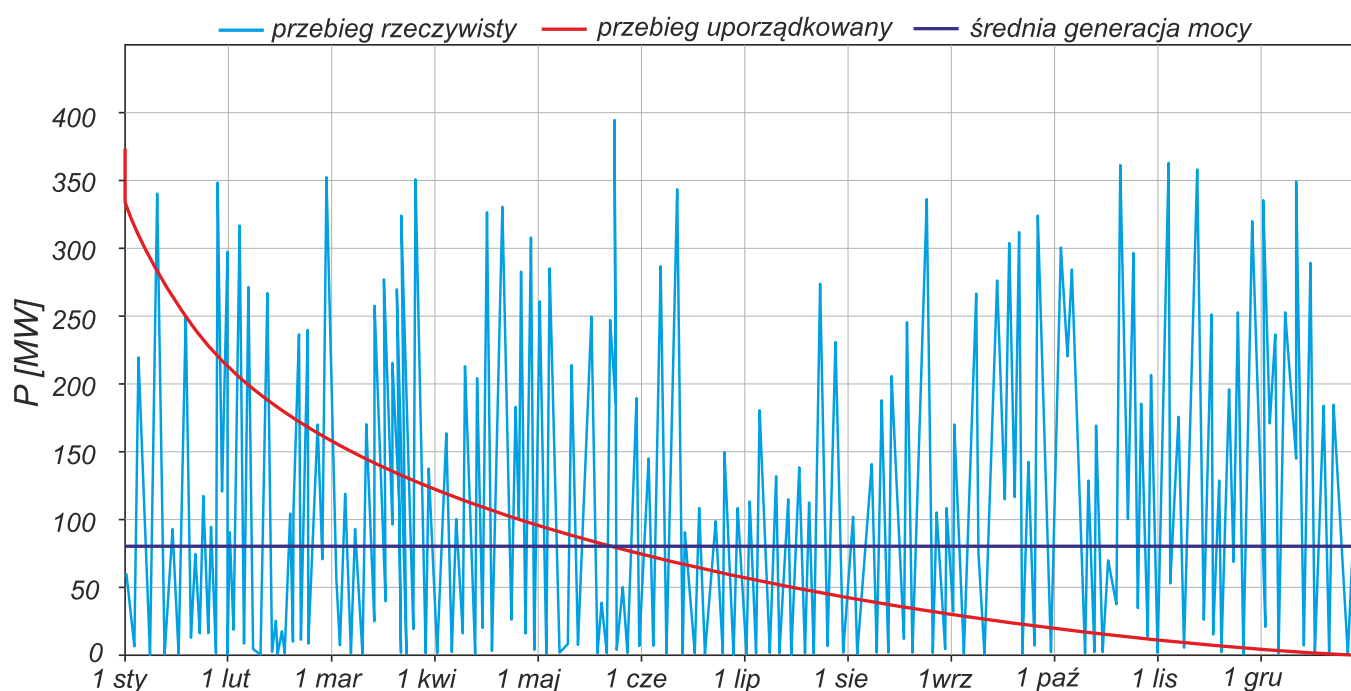
Rys. 1. Roczna zmienność mocy, wg. Prof. Lubośnego, 11 polskich farm wiatrowych o mocy zainstalowanej 455,5 MW
