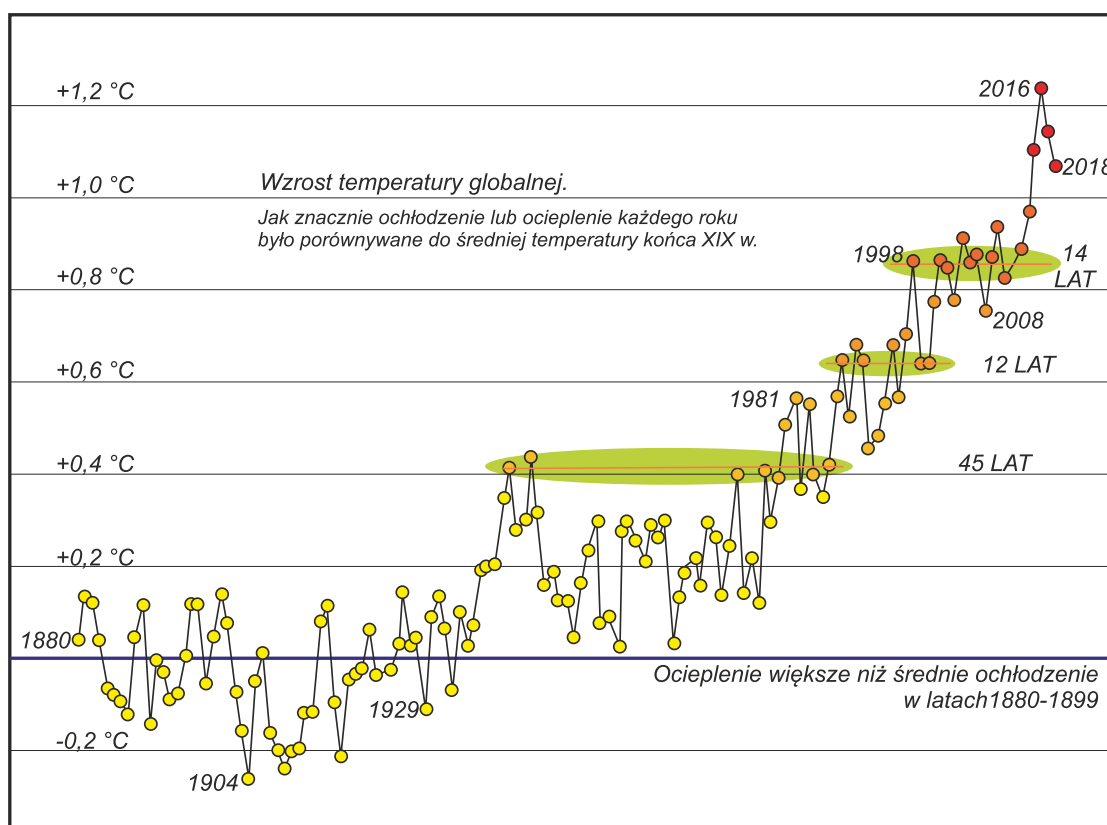
Rys. 3. Zmiany średniej temperatury Ziemi wg. NASA
