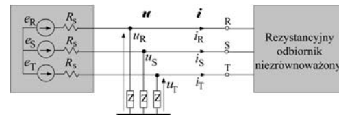
Rys. 4. Obwód trójfazowy z rezystancyjnym niezrównoważonym odbiornikiem Fig. 4. Three-phase system with resistive unbalanced load
