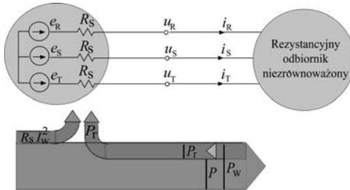
Rys. 6. Diagram przepływu energii w obwodzie rezystancyjnym z odbiornikiem niezrównoważonym
