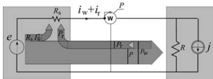
Rys. 2. Diagram przepływu energii w obwodzie z odbiornikiem rezystancyjnym generującym harmonicznyc
