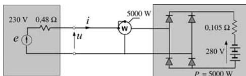
Rys. 3. Obwód z idealnym prostownikiem ładującym baterię akumulatorów Fig. 3. Circuit with an ideal battery charger
